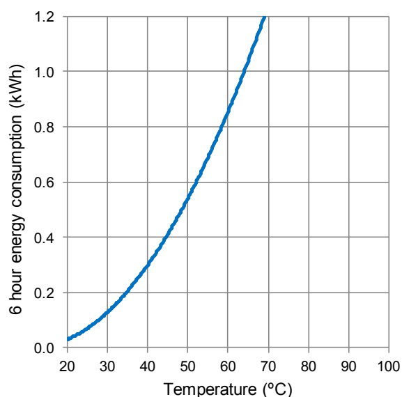
Without lid
