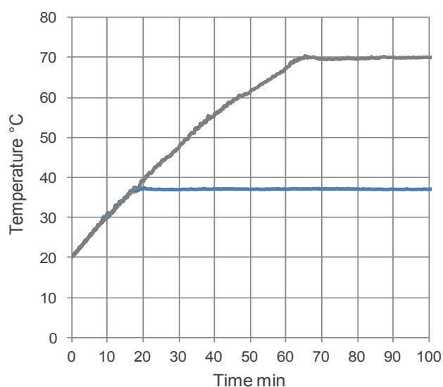
Without lid
