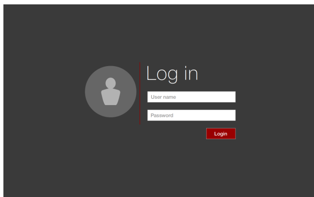
Fig. 28: Login screen
